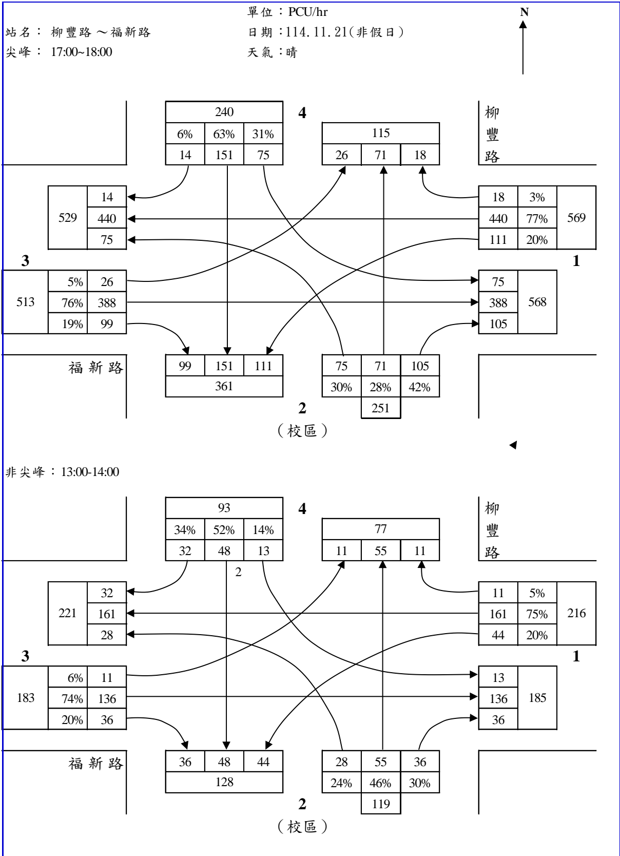
圖 3 柳豐路~福新路路口轉向交通量示意圖(非假日)
