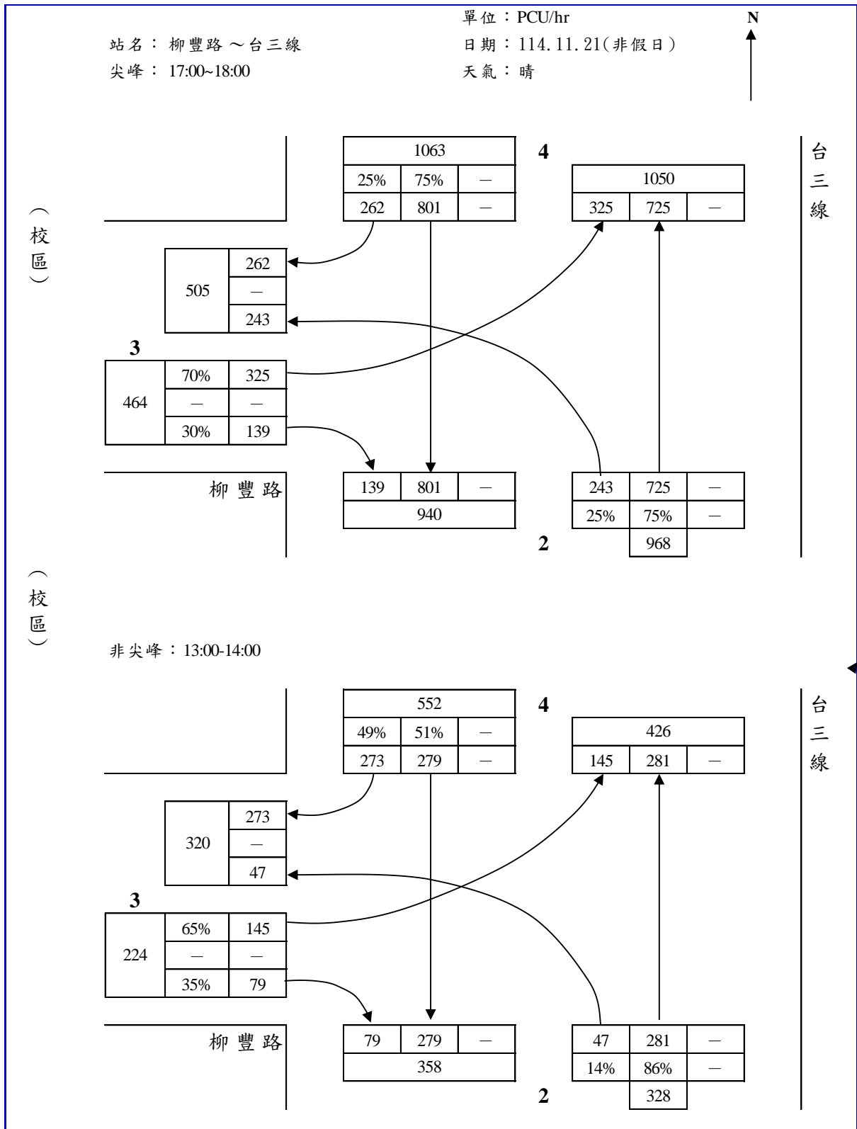
圖 1 柳豐路~台三線路口轉向交通量示意圖(非假日)
