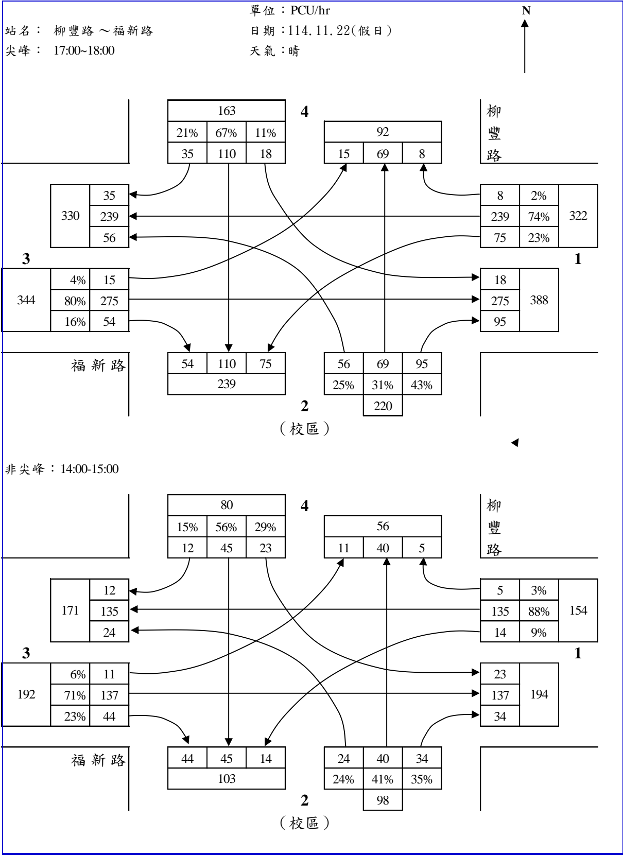
圖 4 柳豐路~福新路路口轉向交通量示意圖(假日)
