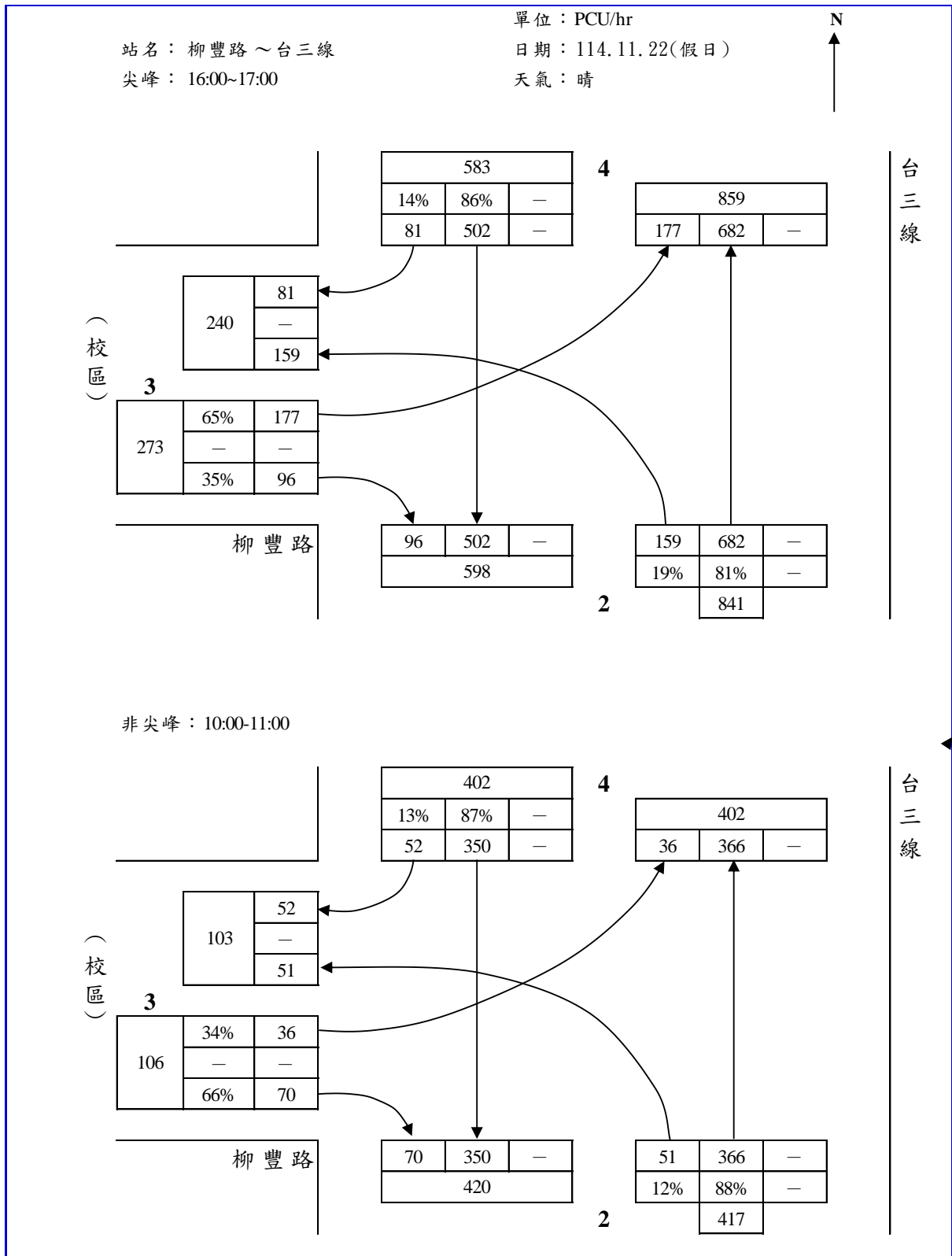
圖 2 柳豐路~台三線路口轉向交通量示意圖(假日)
